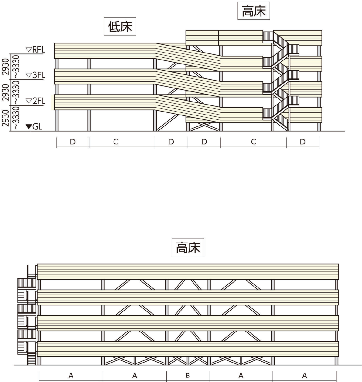
立面図
