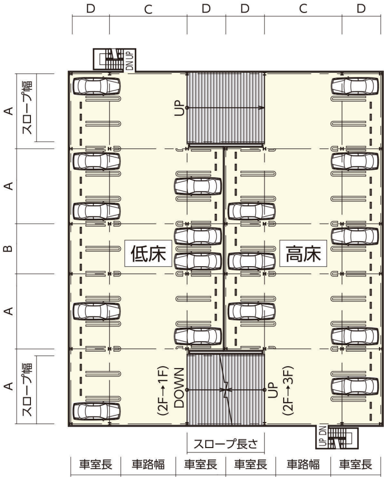
平面図
