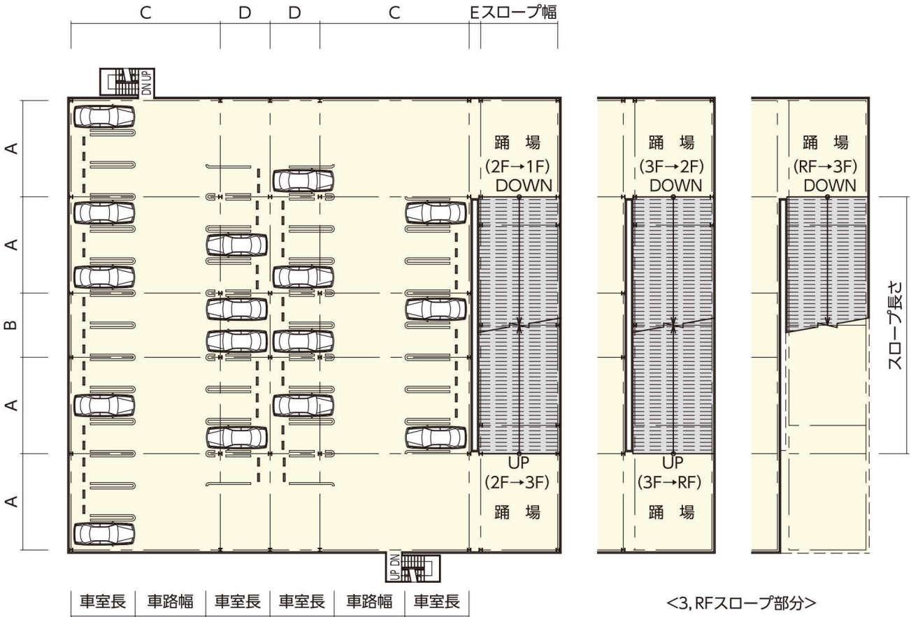
平面図
