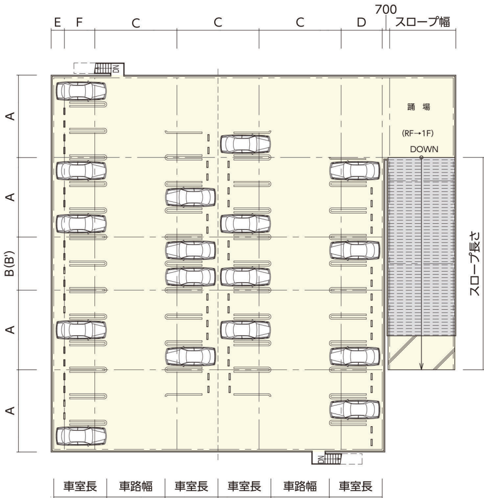
平面図
