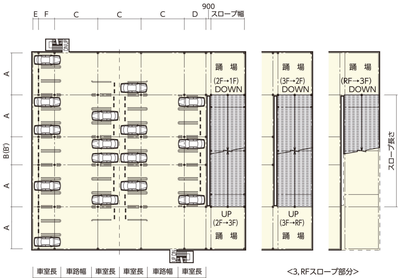
平面図
