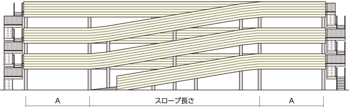
立面図
