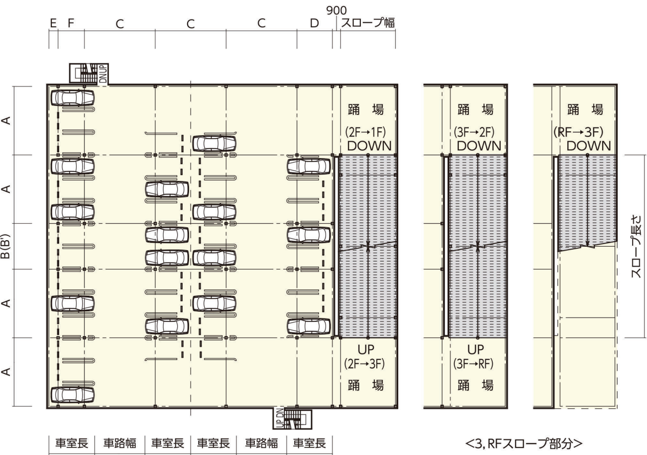
平面図
