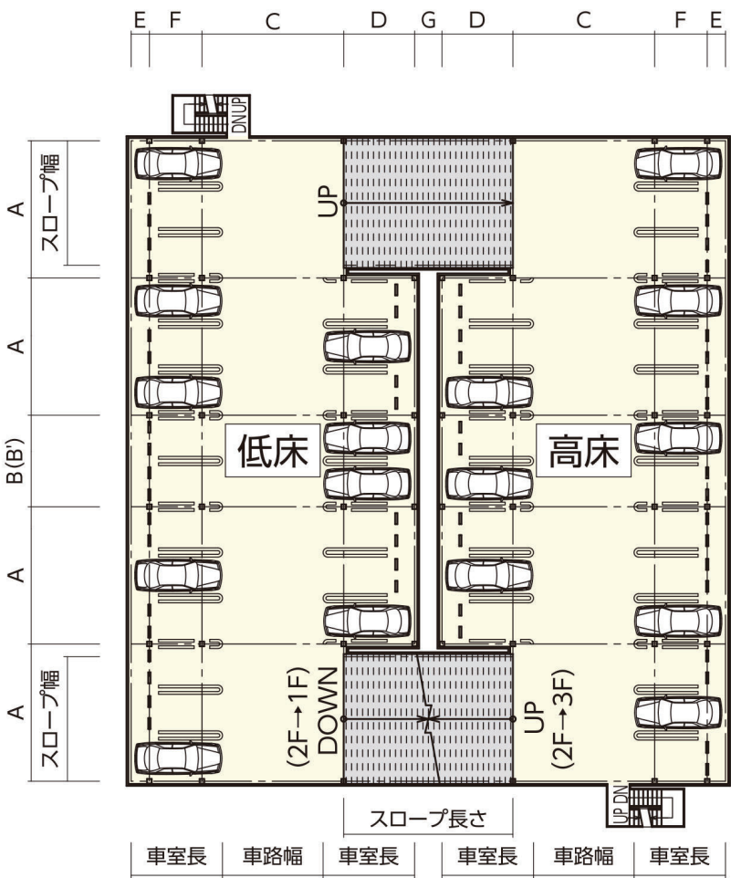
平面図
