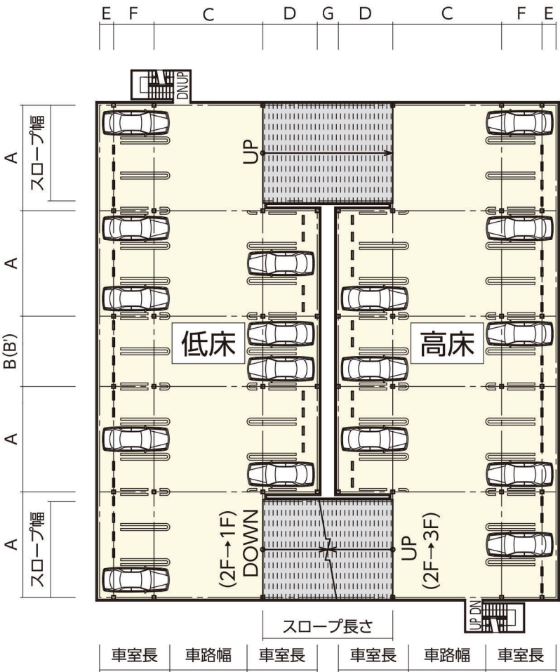
平面図
