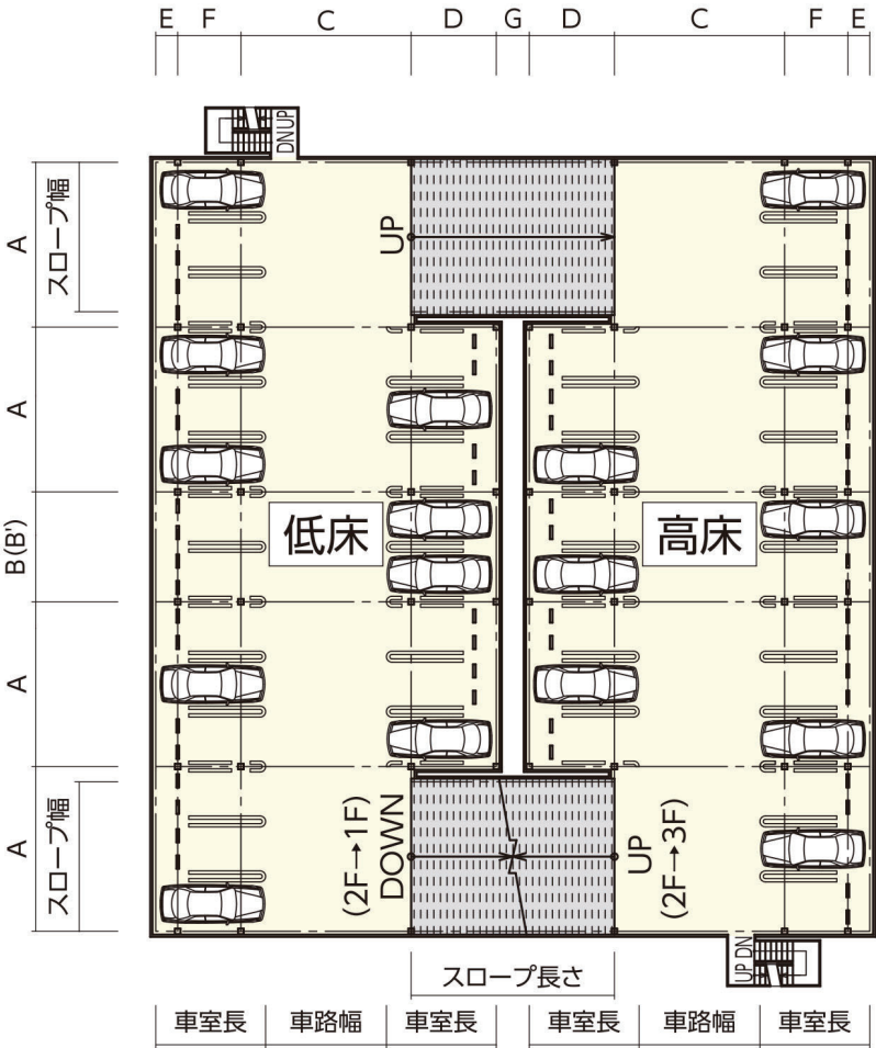
<2F平面図:NC-3N／NC-3NS型>
