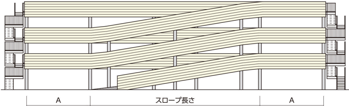
立面図
