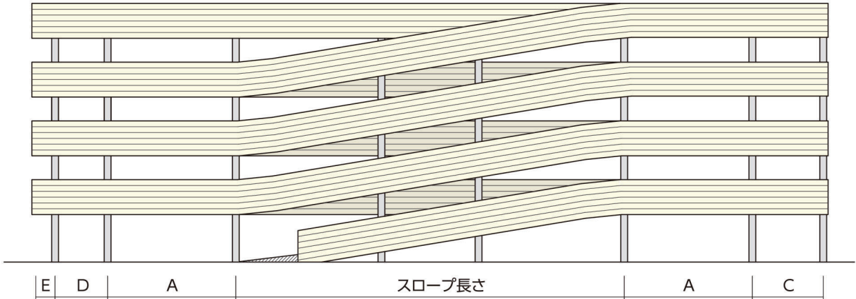
立面図
