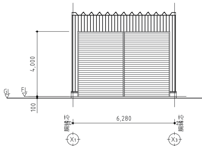
Y1 立面図
