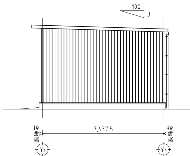
X3 立面図
